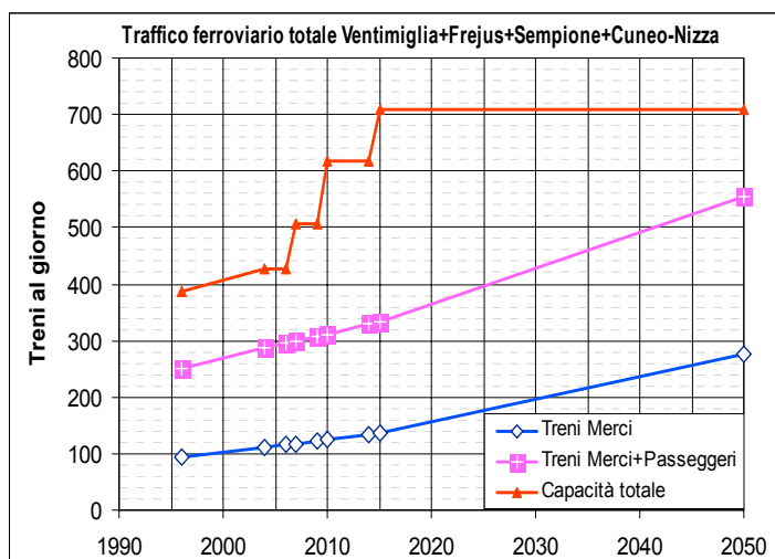
Fig. 4.3-1 Potenziamento To-Modane e Cuneo-Nizza
